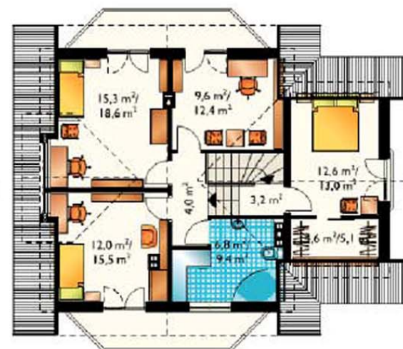
МАНСАРДА
