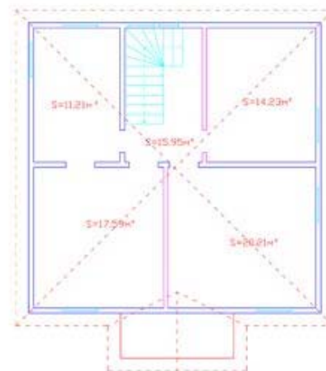
План второго этажа
